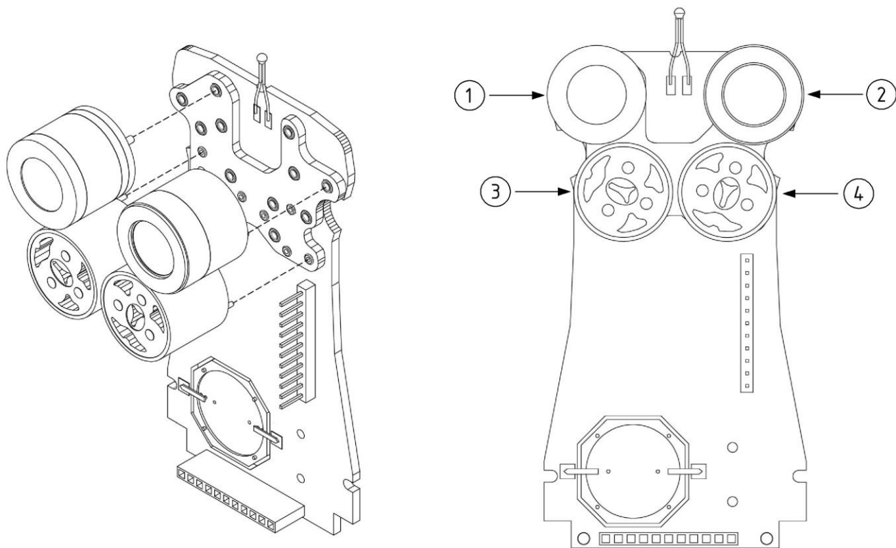
Рисунок 2. Расположение датчиков
